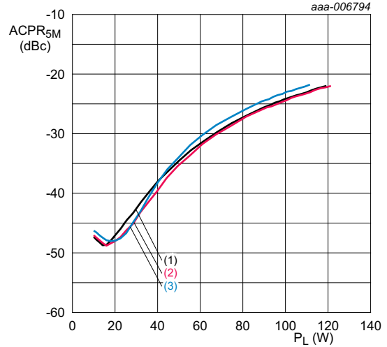
V_{DS} = 28\text{ V} ; I_{Dq} = 1600\text{ mA} ; f = 5\text{ MHz} ; \delta = 46\% . (1) f = 1810\text{ MHz} (2) f = 1843\text{ MHz} (3) f = 1877.5\text{ MHz}
