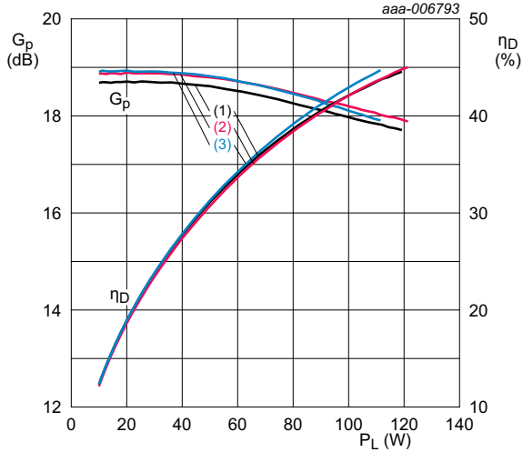
V_{DS} = 28\text{ V} ; I_{Dq} = 1600\text{ mA} ; f = 5\text{ MHz} ; \delta = 46\% . (1) f = 1810\text{ MHz} (2) f = 1843\text{ MHz} (3) f = 1877.5\text{ MHz}
