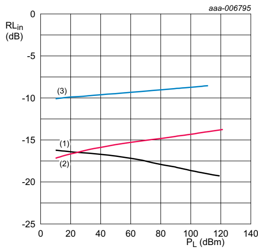
V_{DS} = 28\text{ V} ; I_{Dq} = 1600\text{ mA} ; f = 5\text{ MHz} ; \delta = 46\% . (1) f = 1810\text{ MHz} (2) f = 1843\text{ MHz} (3) f = 1877.5\text{ MHz}
